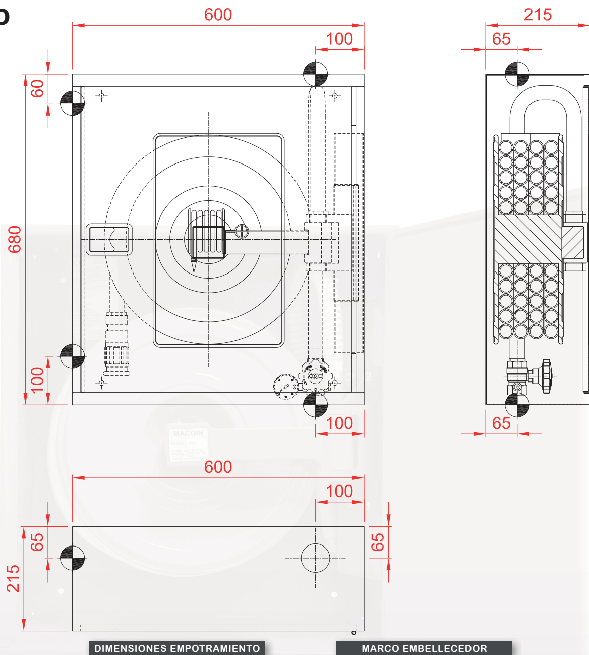
DIMENSIONES EMPOTRAMIENTO
