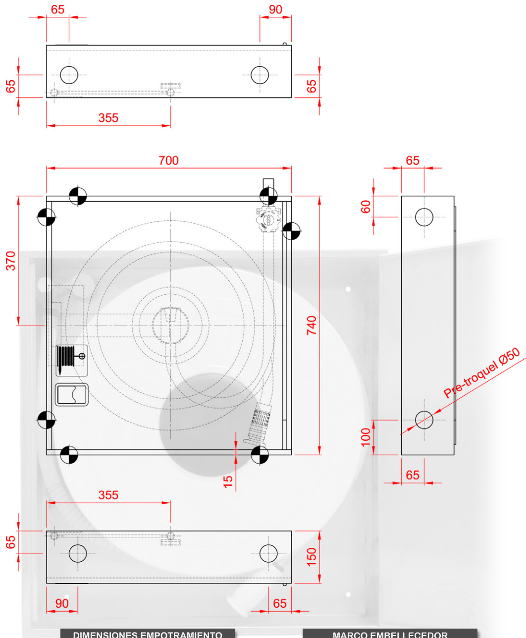
DIMENSIONES EMPOTRAMIENTO
