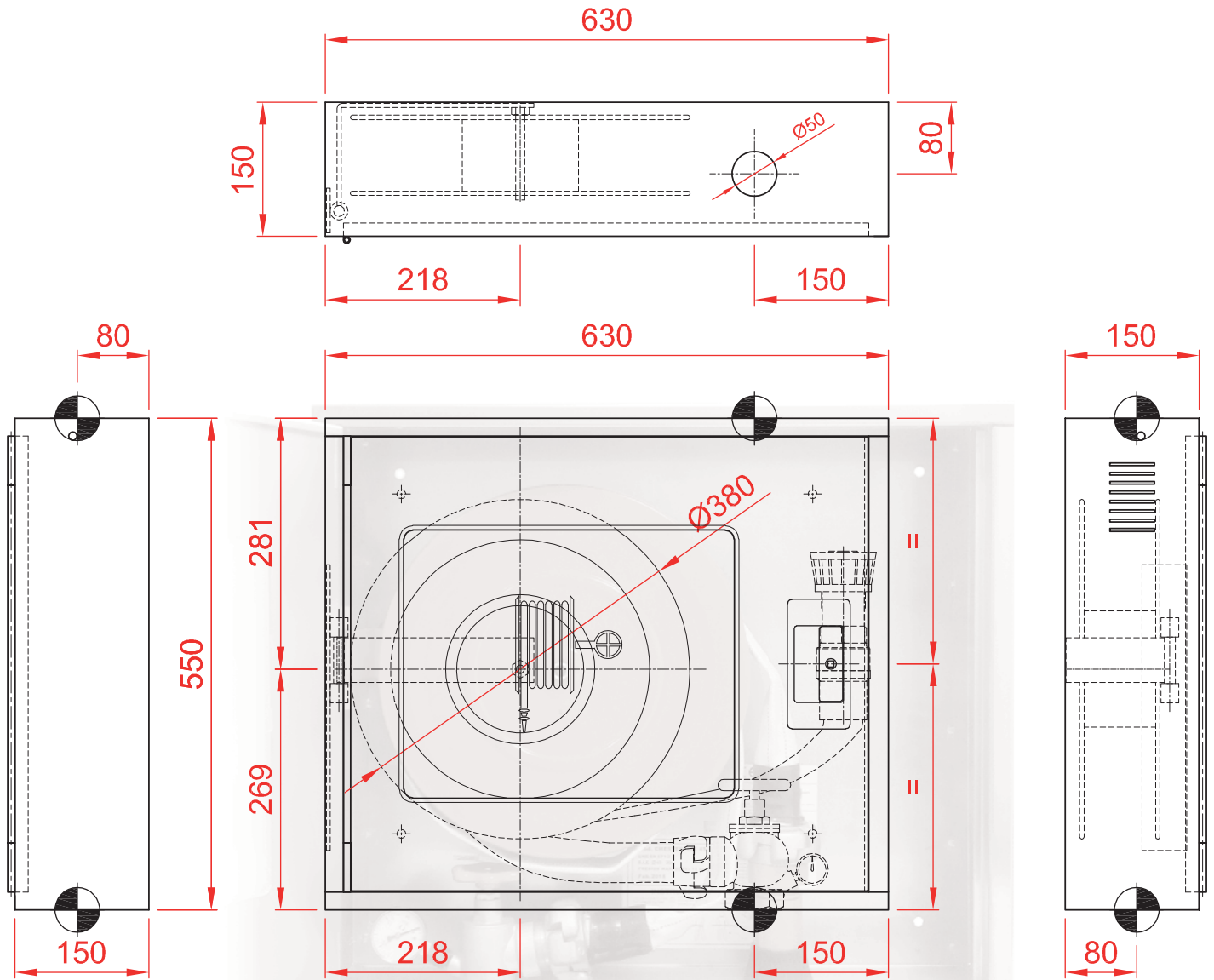
DIMENSIONES EMPOTRAMIENTO
