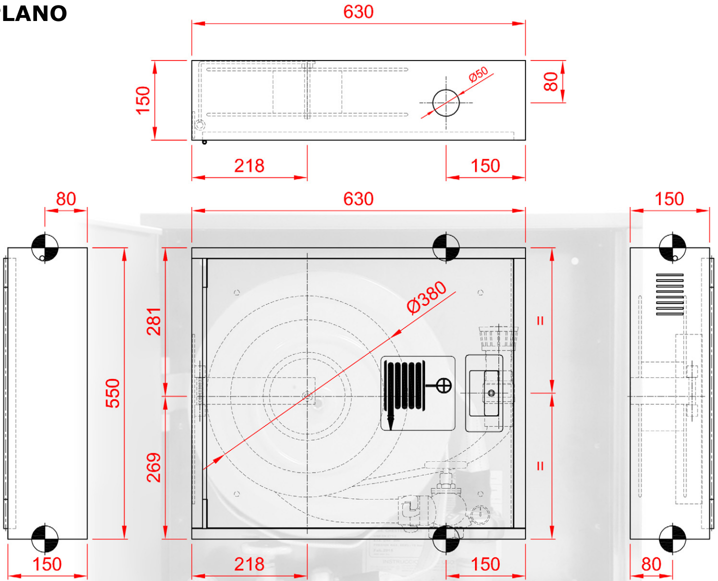
DIMENSIONES EMPOTRAMIENTO
