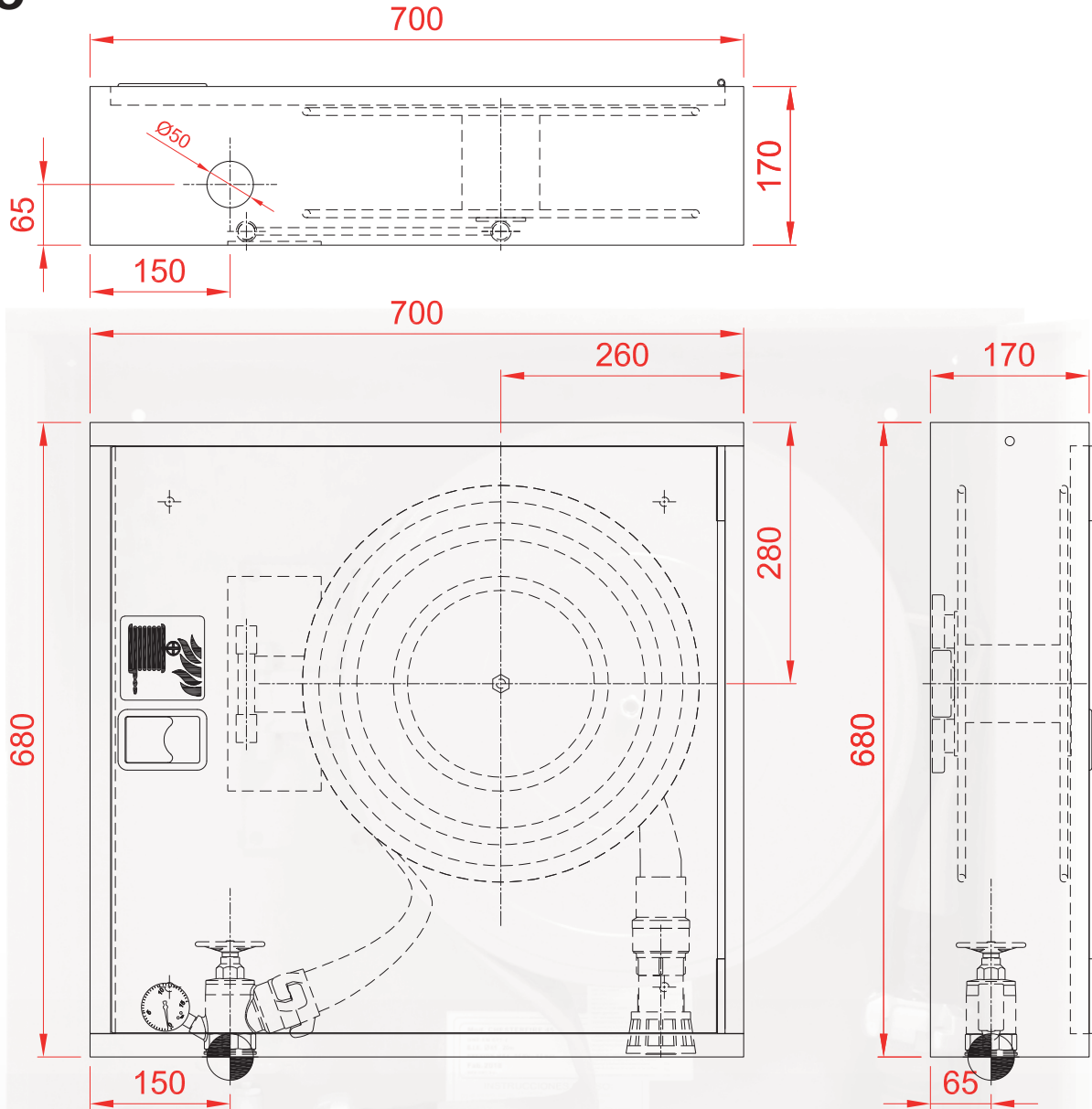
DIMENSIONES EMPOTRAMIENTO
