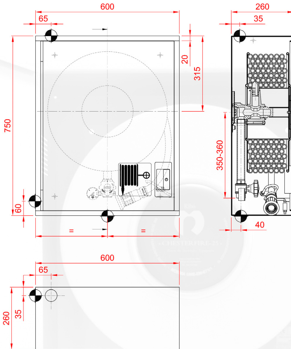
DIMENSIONES EMPOTRAMIENTO
