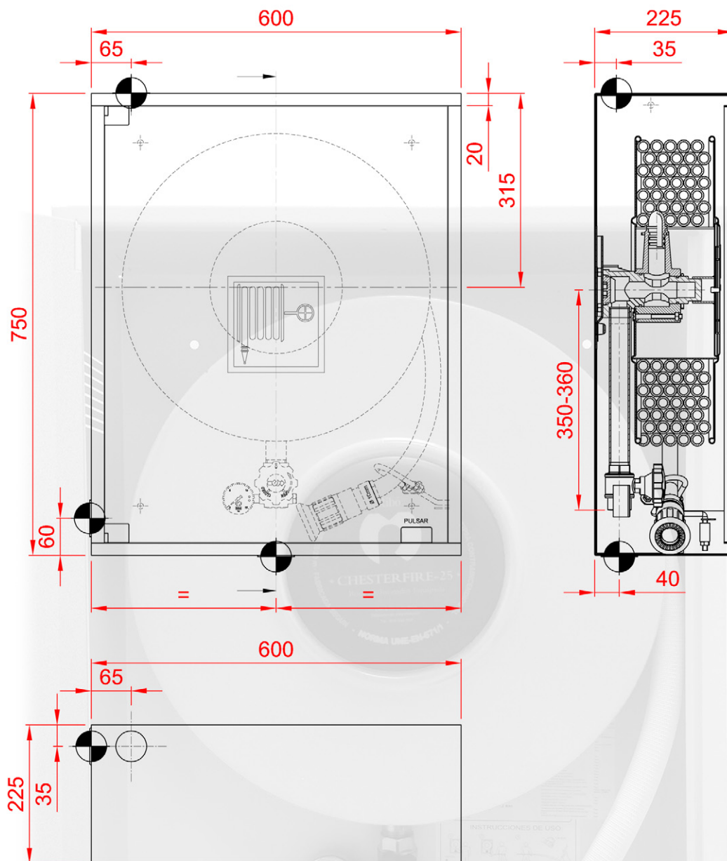
DIMENSIONES EMPOTRAMIENTO
