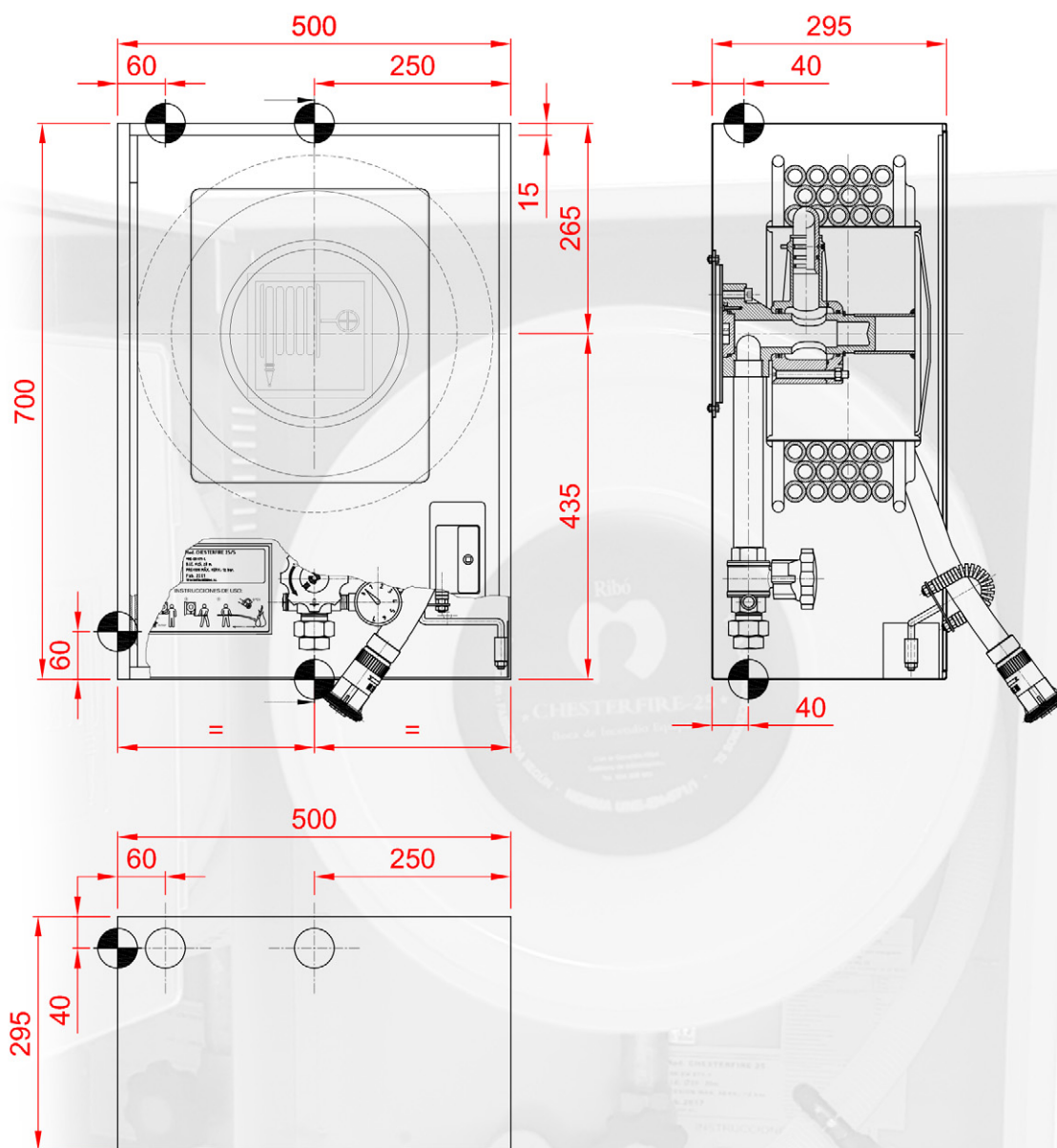
DIMENSIONES EMPOTRAMIENTO
