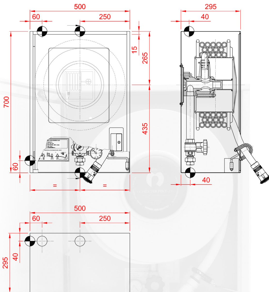
DIMENSIONES EMPOTRAMIENTO
