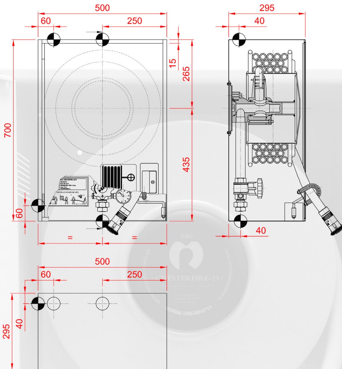
DIMENSIONES EMPOTRAMIENTO
