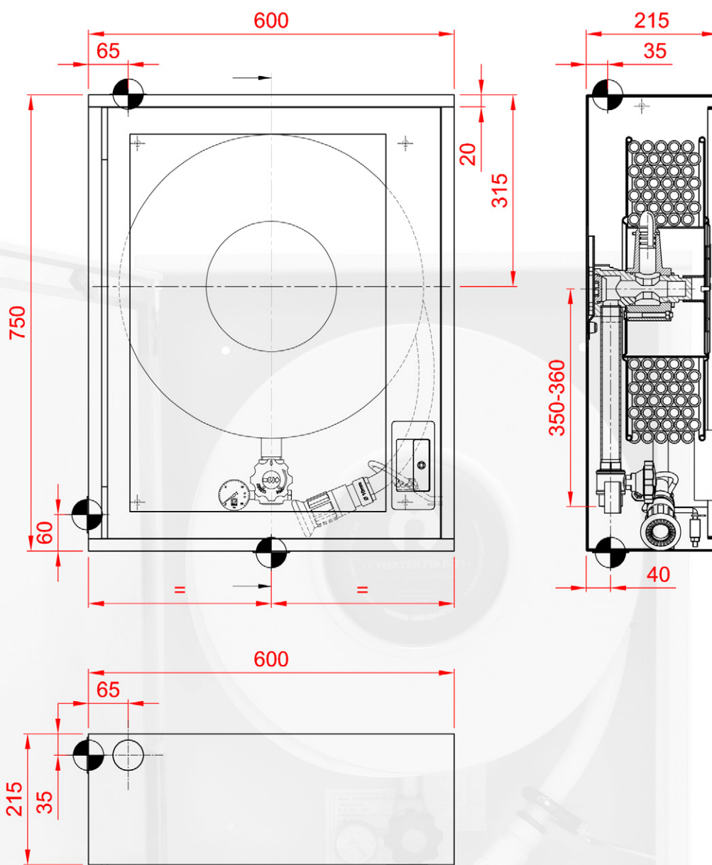
DIMENSIONES EMPOTRAMIENTO
