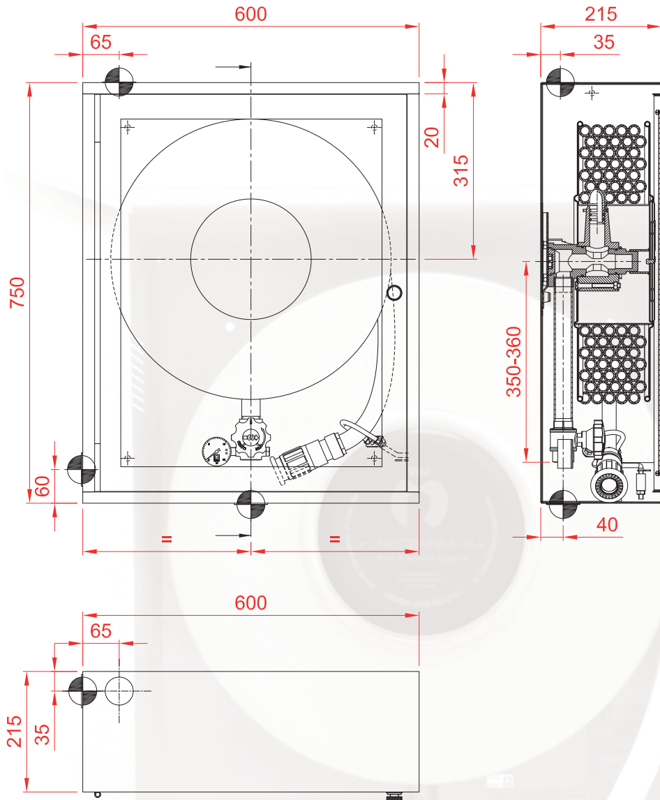
DIMENSIONES EMPOTRAMIENTO
