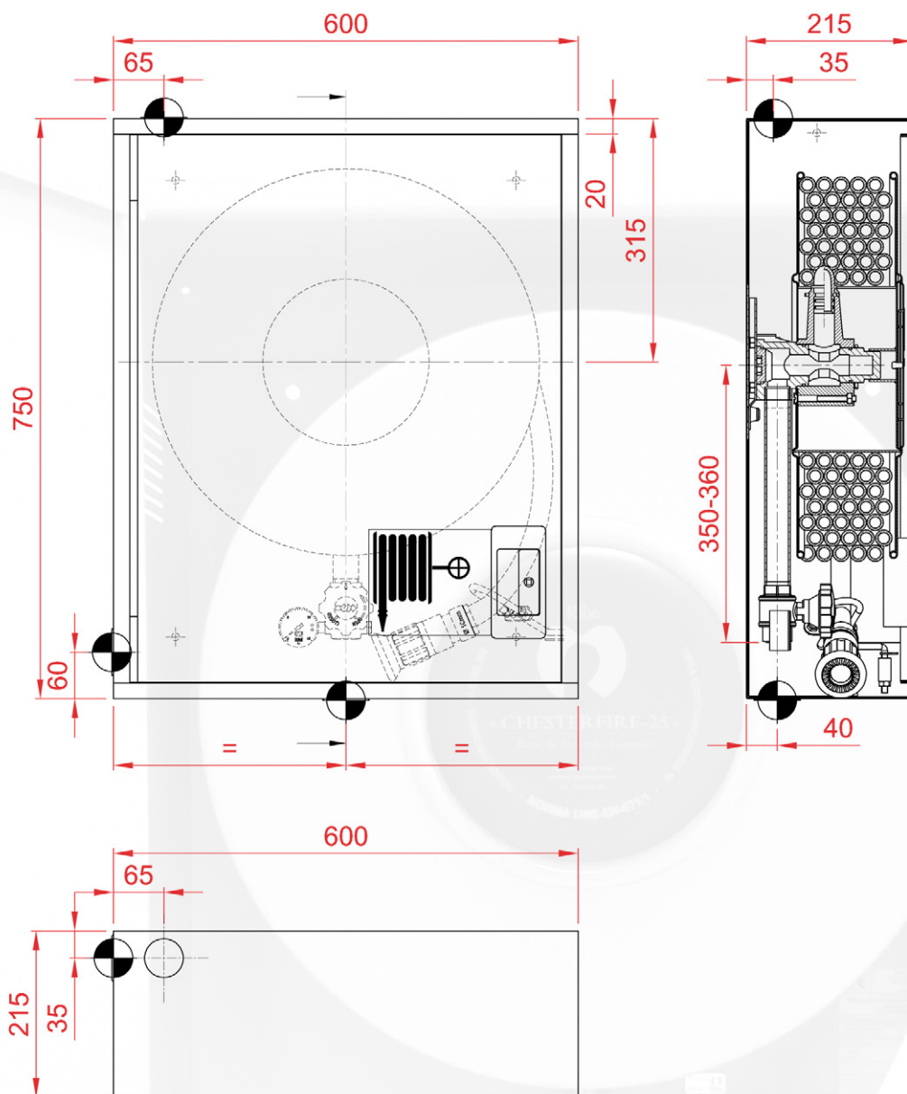
DIMENSIONES EMPOTRAMIENTO
