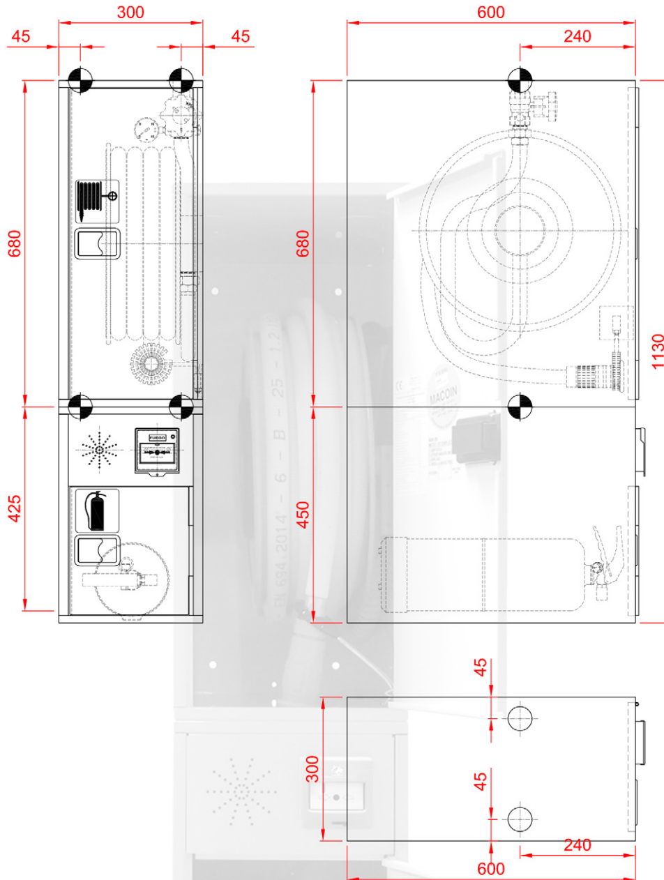
DIMENSIONES EMPOTRAMIENTO
