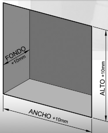
DIMENSIONES EMPOTRAMIENTO
