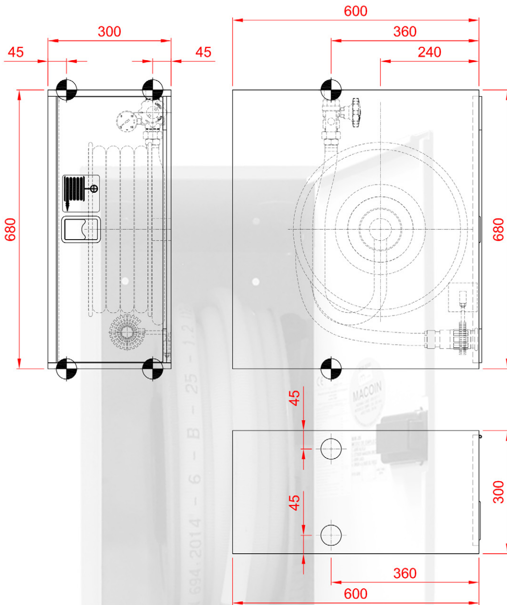
DIMENSIONES EMPOTRAMIENTO
