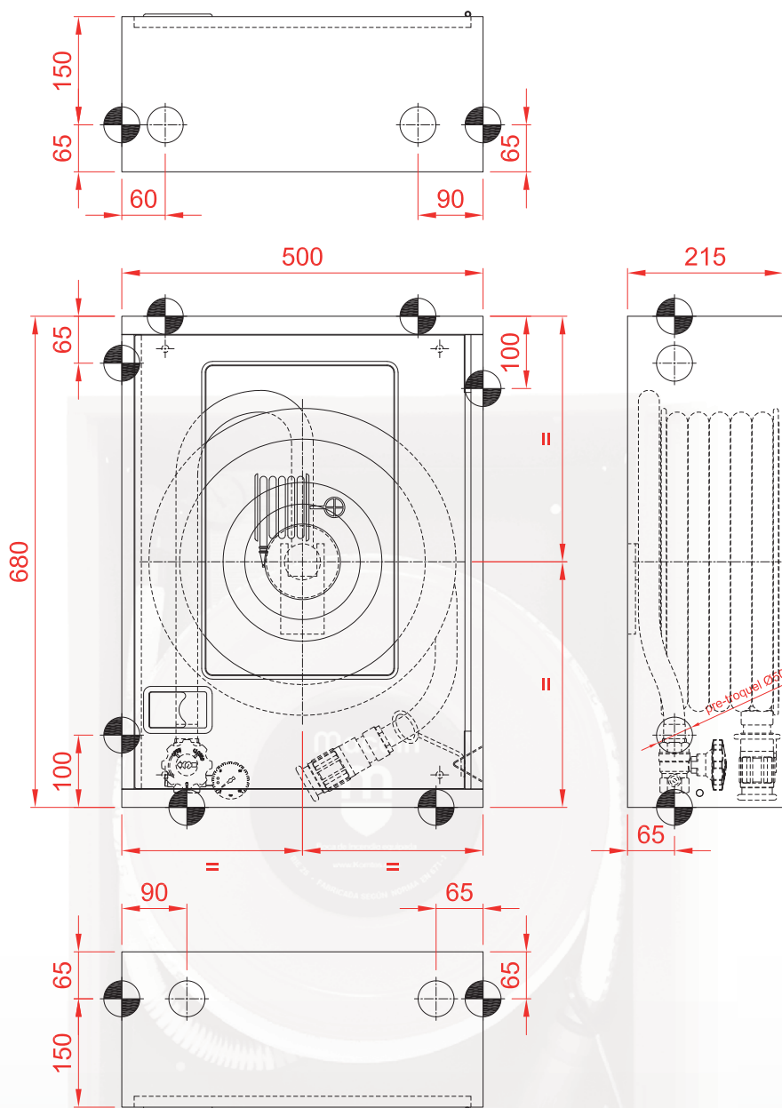
DIMENSIONES EMPOTRAMIENTO
