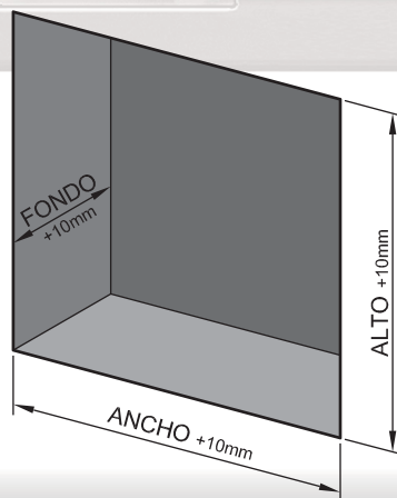
DIMENSIONES EMPOTRAMIENTO
