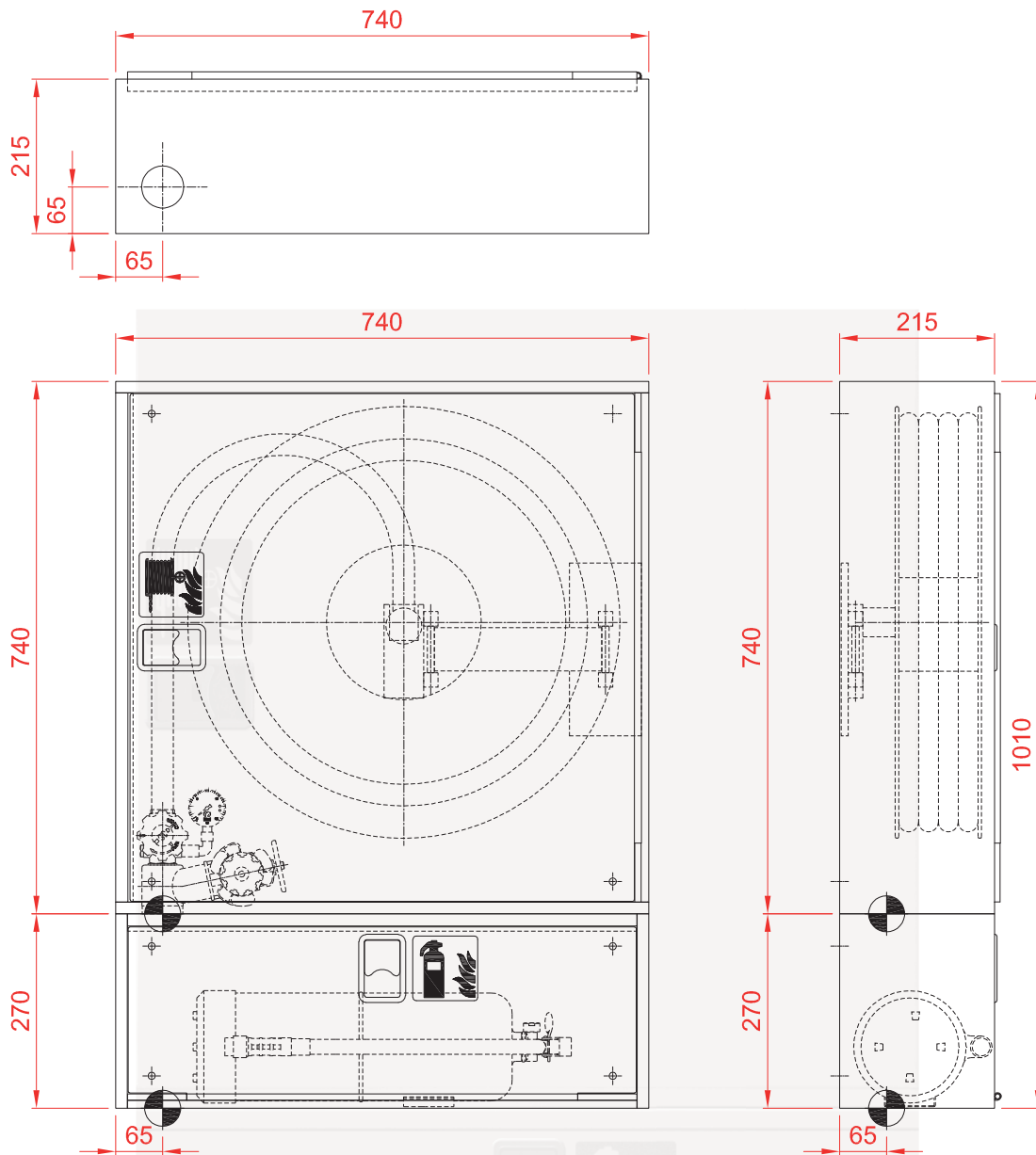
DIMENSIONES EMPOTRAMIENTO
