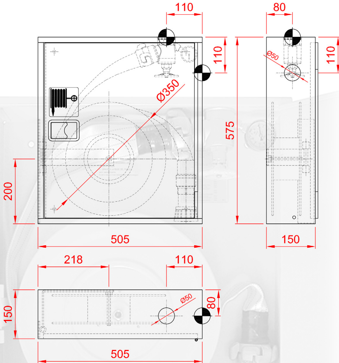
DIMENSIONES EMPOTRAMIENTO
