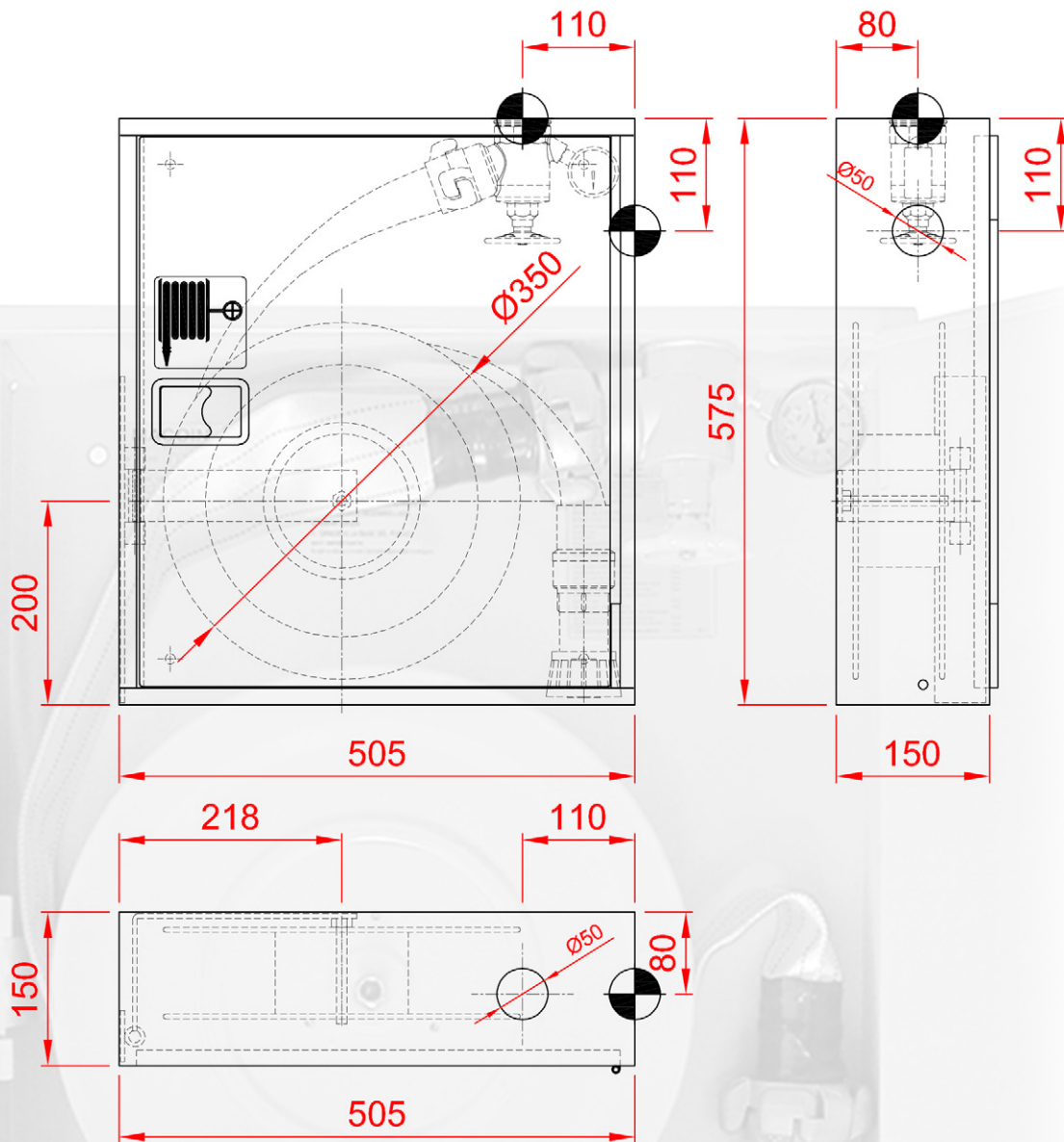
DIMENSIONES EMPOTRAMIENTO
