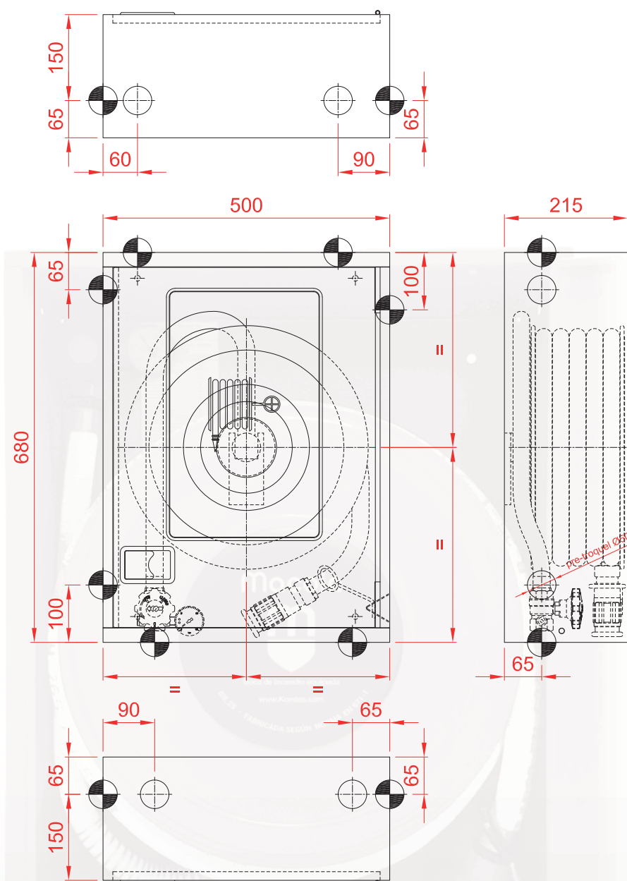
DIMENSIONES EMPOTRAMIENTO
